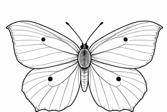
latolistek cytrynek
