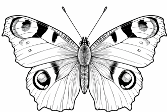
rusatka pawik
