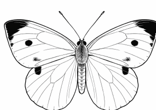
bielinek kapustnik
